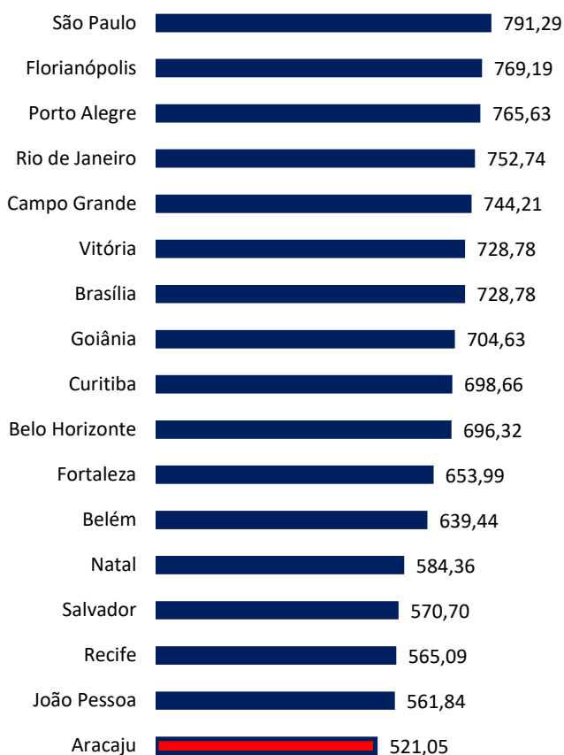
Gráfico 2: Custo Mensal da Cesta Básica das capitais (R$) – Dezembro/2022
