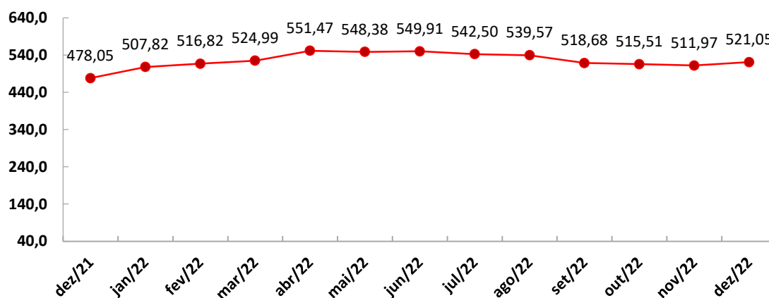
Gráfico 1: Custo Mensal da Cesta Básica (R$) - Aracaju – dezembro/2021 – dezembro/2022
