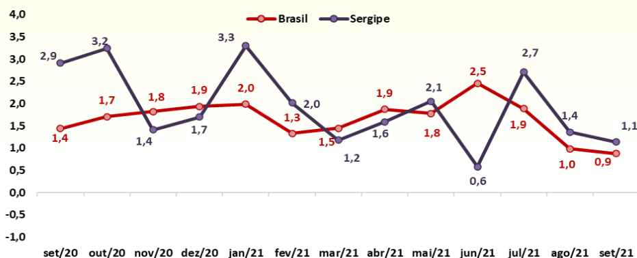
Varição do custo médio por m 2 (%) - Sergipe - Setembro/2020 a Setembro/2021
